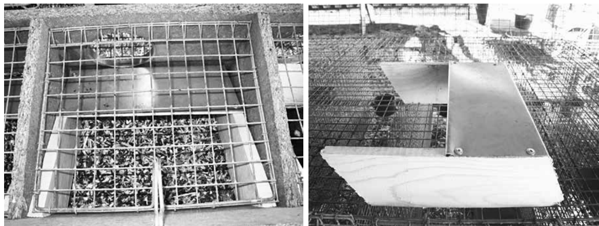
Рис. 3. Ветрозащитная вставка: слева – внешний вид, справа – внутри домика.
