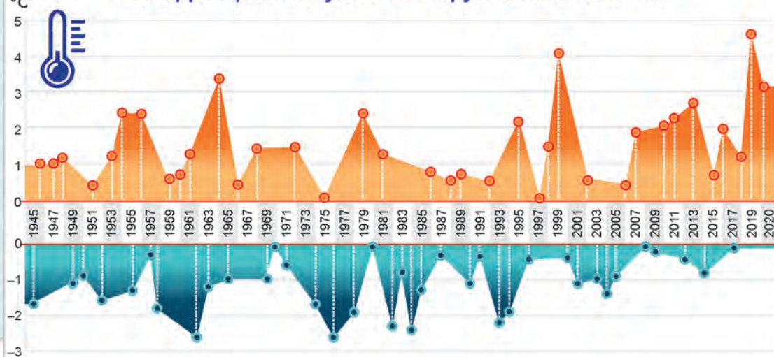
Отклонение средней месячной температуры воздуха июня от климатической нормы (+16,4 °C) по территории Республики Беларусь за 1945–2020 гг.
